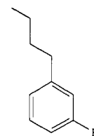
13 : R = H 15 : R = CH 3
